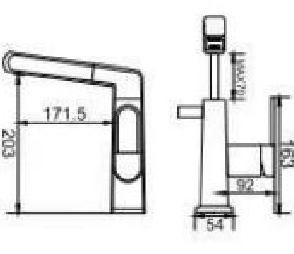
20223 单把抽拉面盆龙头 Pull-out basin faucet 主体材质：铜 /Material: Brass
