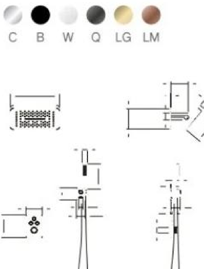
21047 三功能恒温暗装淋浴花洒 3F constanttemperature concealed shower 主体材质：铜 /Material: Brass
