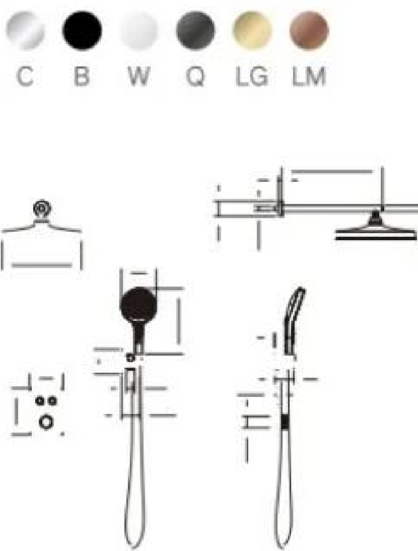
21046 二功能恒温暗装淋浴花洒 2F constanttemperature concealed shower 主体材质：铜 /Material: Brass
