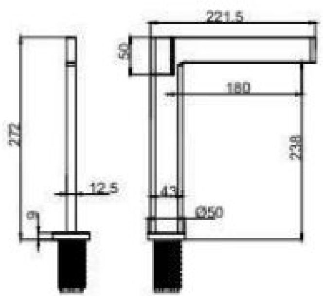
20162 单把面盆龙头 Single handle basin faucet 主体材质：铜 /Material: Brass
