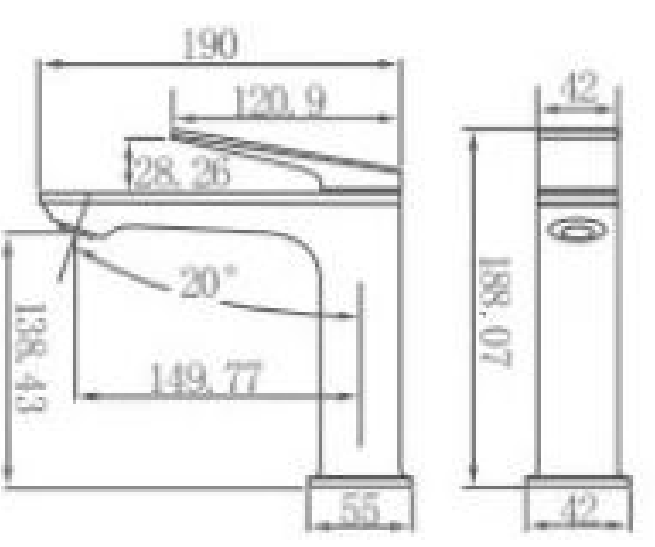
25208 单把面盆龙头 Single handle basin faucet 主体材质：铜 /Material: Brass
