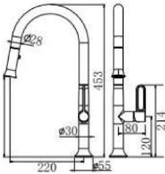
20224 单把抽拉厨房龙头 Pull-out kitchen mixer 主体材质：铜 /Material: Brass
