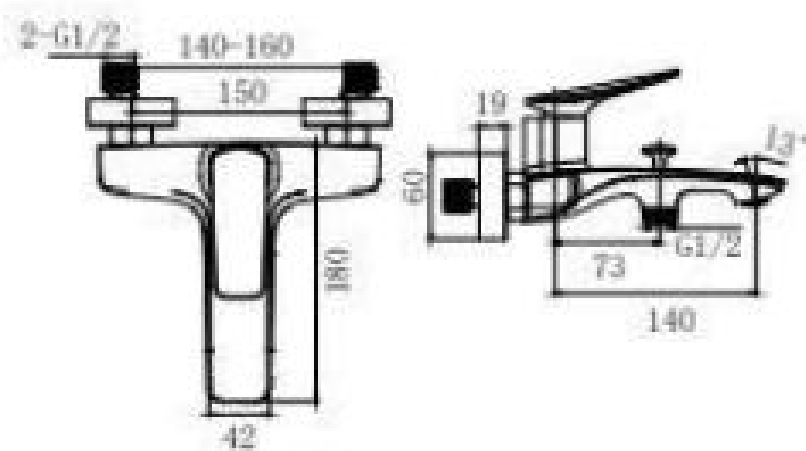
20107 单把浴缸龙头 Single handle Bathtub Faucet 主体材质：铜 /Material: Brass
