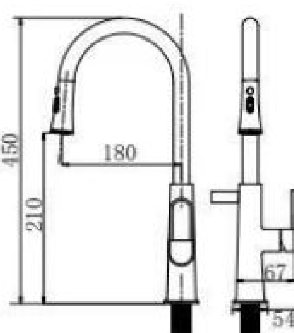
20225 单把抽拉厨房龙头 Pull-out kitchen mixer 主体材质：铜 /Material: Brass
