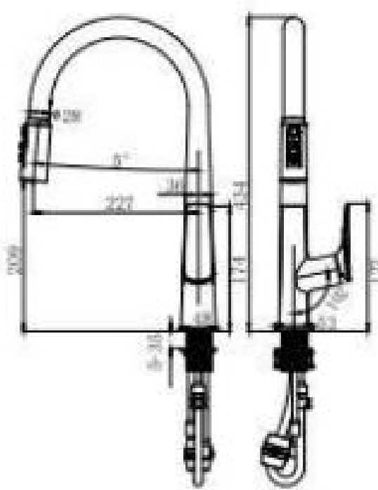
20106 单把抽拉厨房龙头 Pull-out kitchen mixer 主体材质：铜 /Material: Brass
