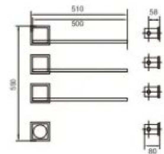
27015 电热毛巾架 Electric towel rack 主体材质 :SUS304/Material: SUS304
