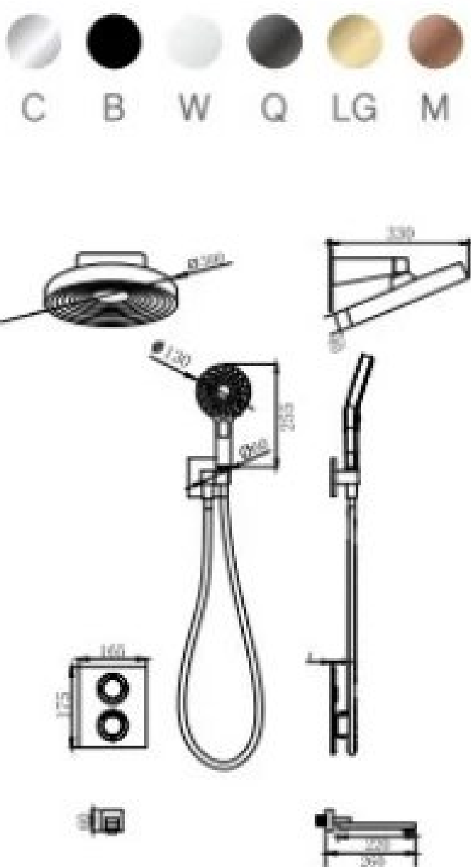
21035 二功能恒温暗装淋浴花洒 2F constanttemperature concealed shower 主体材质：铜 /Material: Brass
