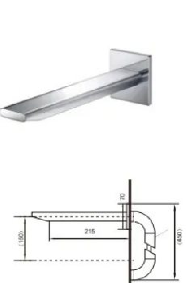
26008 单把面盆龙头 Single handle basin faucet 主体材质：铜 /Material: Bra
