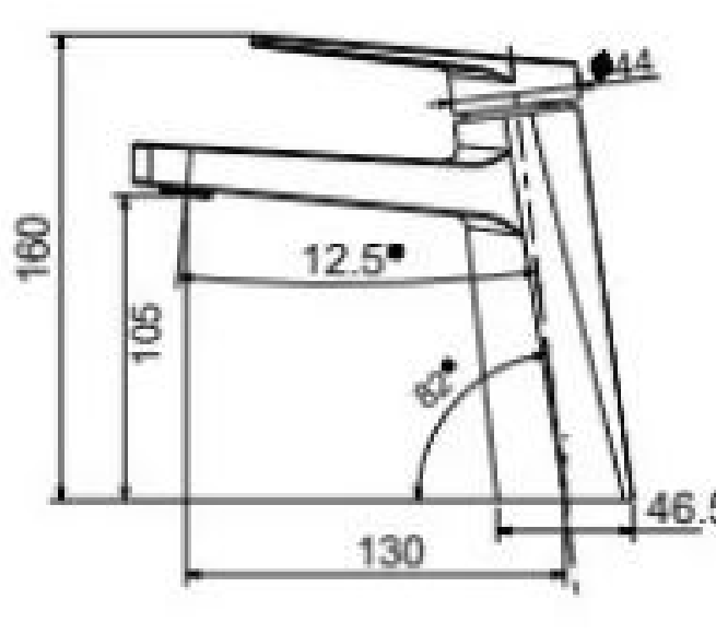
25206 单把面盆龙头 Single handle basin faucet 主体材质：铜 /Material: Brass
