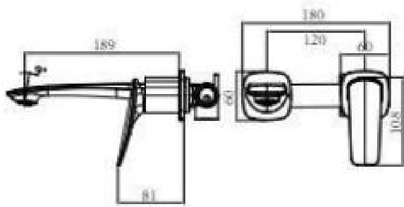
20105 单把入墙面盆龙头 Single handle basin faucet 主体材质：铜 /Material: Brass
