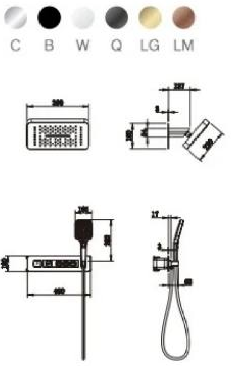
21045 三功能恒温暗装淋浴花洒 3F constanttemperature concealed shower 主体材质：铜 /Material: Brass
