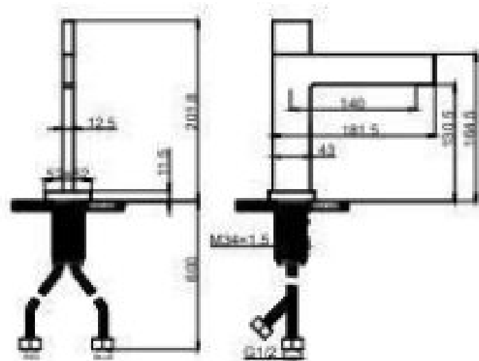
20163 单把面盆龙头 Single handle basin faucet 主体材质：铜 /Material: Brass
