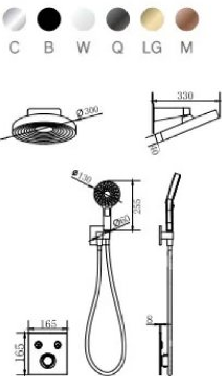
21034 二功能恒温暗装淋浴花洒 2F constanttemperature concealed shower 主体材质：铜 /Material: Brass
