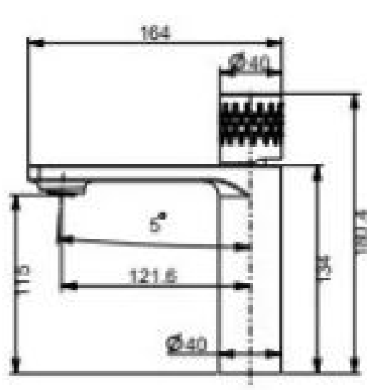
25207 单把面盆龙头 Single handle basin faucet 主体材质：铜 /Material: Brass
