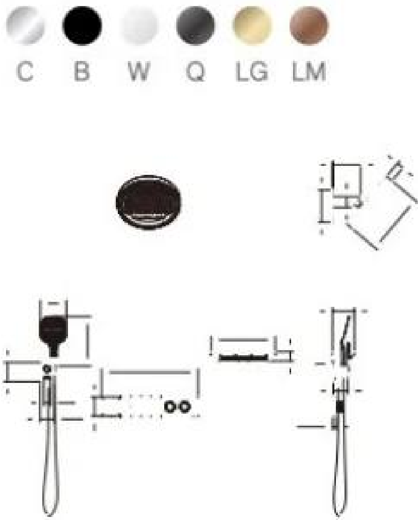
21042 四功能恒温暗装淋浴花洒 4F constanttemperature concealed shower 主体材质：铜 /Material: Brass
