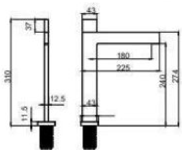
20164 单把面盆龙头 Single handle basin faucet 主体材质：铜 /Material: Brass
