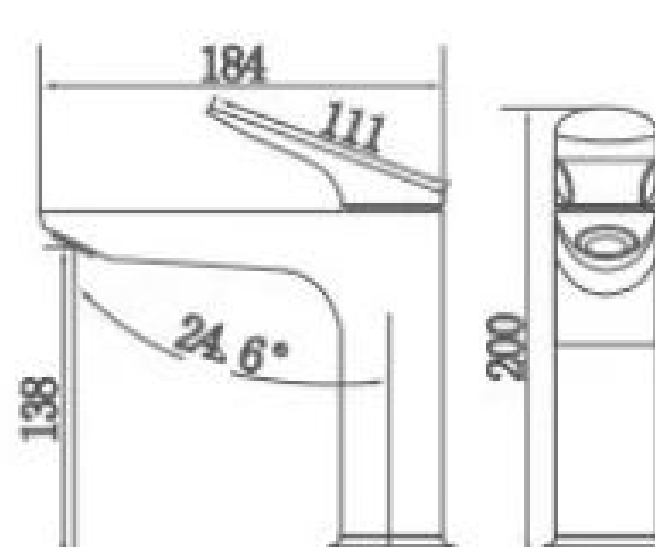
25210 单把面盆龙头 Single handle basin faucet 主体材质：铜 /Material: Brass
