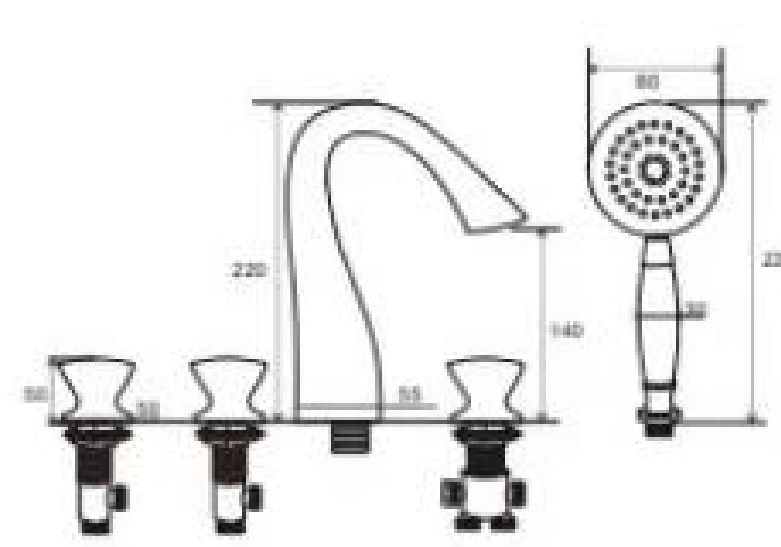
25004 分体浴缸龙头 Single handle Bathtub Faucet 主体材质：铜 /Material: Brass
