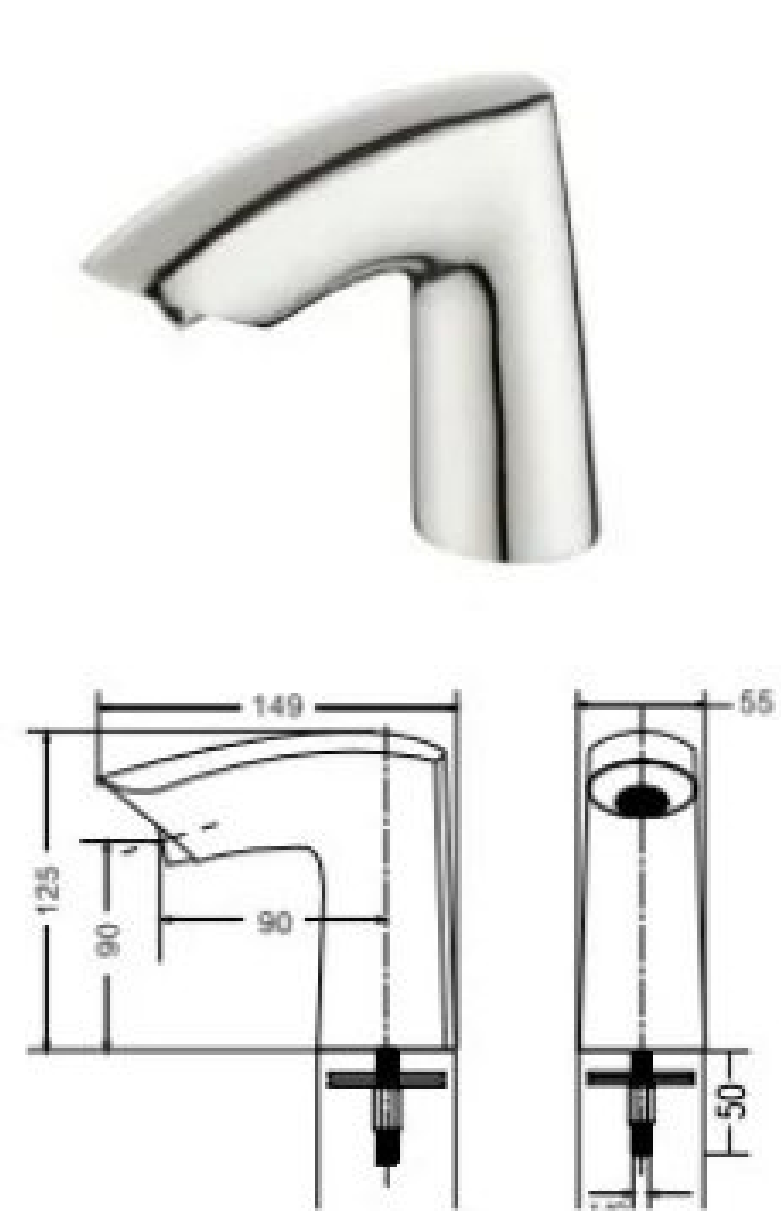
26001 单把面盆龙头 Single handle basin faucet 主体材质：铜 /Material: Brass
