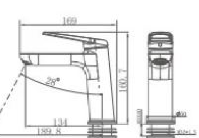
25211 单把面盆龙头 Single handle basin faucet 主体材质：铜 /Material: Brass
