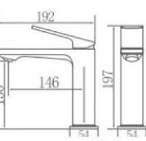
25209 单把面盆龙头 Single handle basin faucet 主体材质：铜 /Material: Brass
