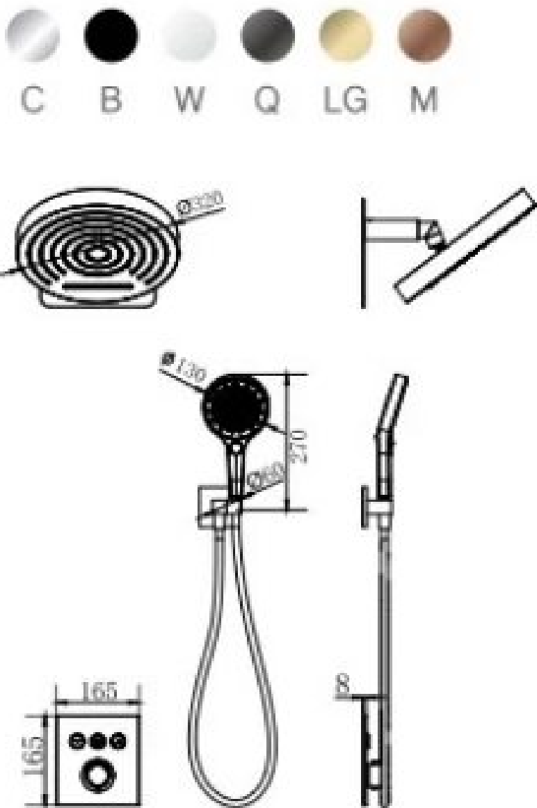
21033 二功能恒温暗装淋浴花洒 2F constanttemperature concealed shower 主体材质：铜 /Material: Brass
