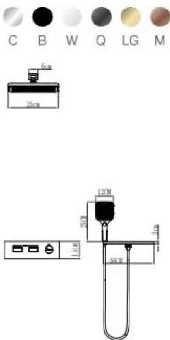
21025 二功能恒温暗装淋浴花洒 2F constanttemperature concealed shower 主体材质：铜 /Material: Brass
