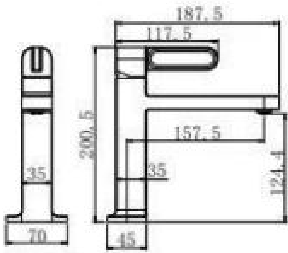
20222 单把面盆龙头 Single handle basin faucet 主体材质：铜 /Material: Brass
