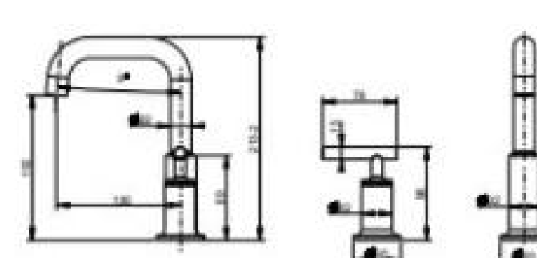
25003 双把分体面盆龙头 Single handle basin faucet 主体材质：铜 /Material: Brass
