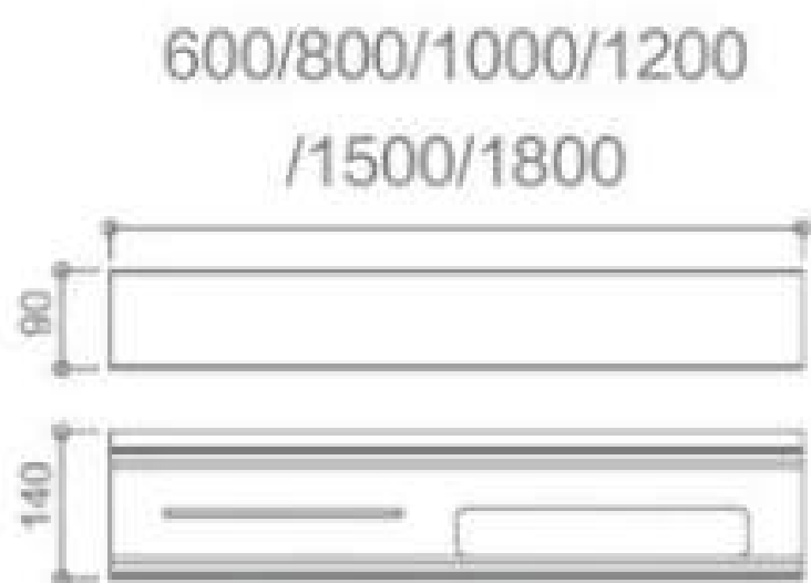
27102 多功能置物架 Multi functional storage rack 主体材质 : 太空铝 /Material: Space aluminum
