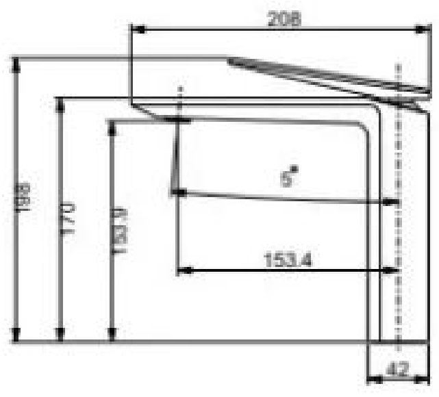
25205 单把面盆龙头 Single handle basin faucet 主体材质：铜 /Material: Brass
