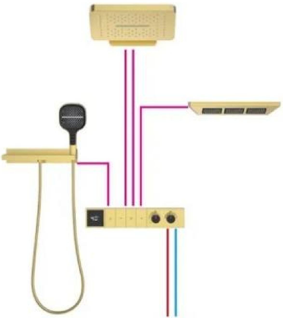
21042 四功能恒温暗装淋浴花洒 4F constanttemperature concealed shower 主体材质：铜 /Material: Brass
