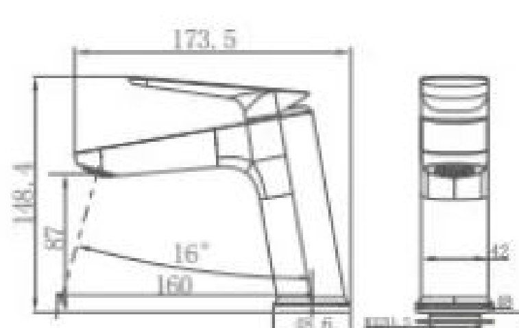
25212 单把面盆龙头 Single handle basin faucet 主体材质：铜 /Material: Brass
