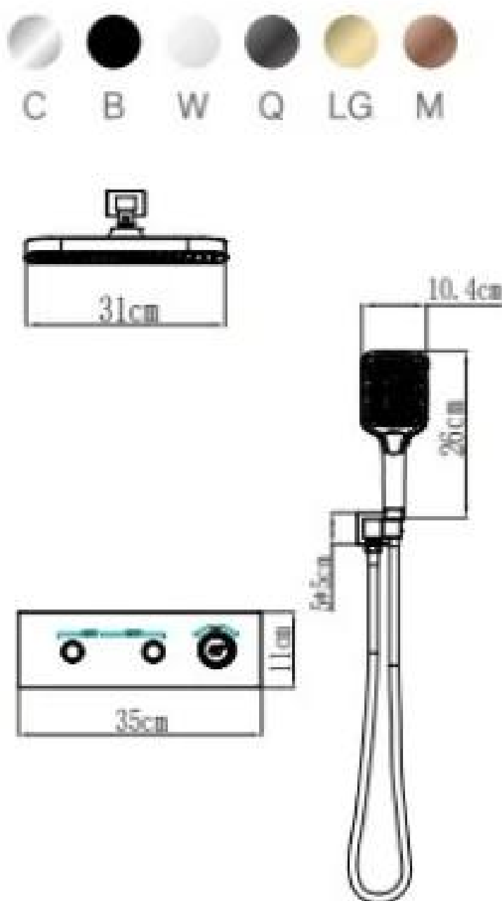
21026 二功能恒温暗装淋浴花洒 2F constanttemperature concealed shower 主体材质：铜 /Material: Brass
