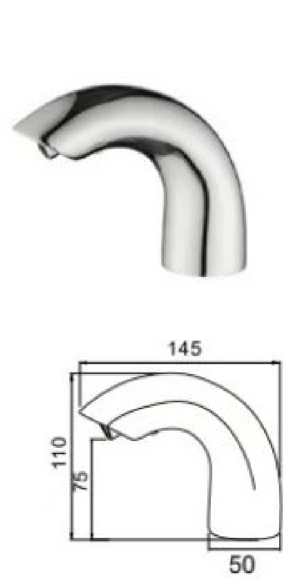
26001 单把面盆龙头 Single handle basin faucet 主体材质：铜 /Material: Brass
