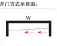
HF-053 产品类型：屏风三联动门 玻璃厚度：8 / 10mm 五金材质：SUS304不锈钢 颜色：镜光 可选：钛金 / 玫瑰金 非标范围：W1200-1500mm H 1900-2200mm
