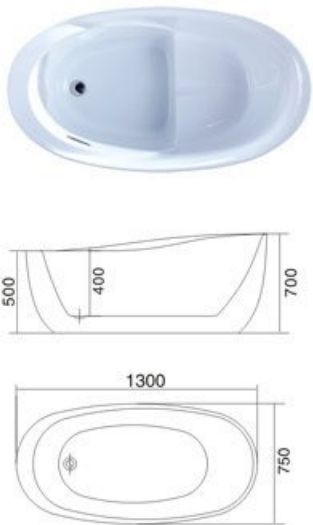
Model: H-7091 SIZE: 1300x750x700mm 可选不带座位
