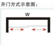
HF-034 产品类型：屏风双活动门 玻璃厚度：8 / 10mm 五金材质：SUS304不锈钢 颜色：镜光 可选：钛金 / 玫瑰金 非标范围：W1200-1500mm H 1900-2200mm
