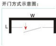
HF-046 产品类型：屏风两固一活 玻璃厚度：8 / 10mm 五金材质：SUS304不锈钢 颜色：镜光 可选：钛金 / 玫瑰金 非标范围：W1200-1500mm H 1900-2200mm
