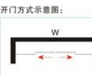
HF-009 产品类型：屏风两固两活 玻璃厚度：8 / 10mm 五金材质：铝材 颜色：亮银 可选：砂银 / 哑银 / 拉丝 非标范围：W800-1500mm H1900-2200mm
