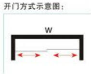
HF-052 产品类型：屏风双活动门 玻璃厚度：8 / 10mm 五金材质：SUS304不锈钢 颜色：镜光 可选：钛金 / 玫瑰金 非标范围：W1200-1500mm H 1900-2200mm
